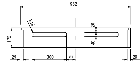
B-B 断面図 S=1/10 (S=1/20)
