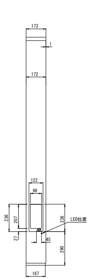
側面図 S=1/10 (S=1/20)
