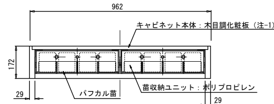
A-A 断面図 S=1/10 (S=1/20)
