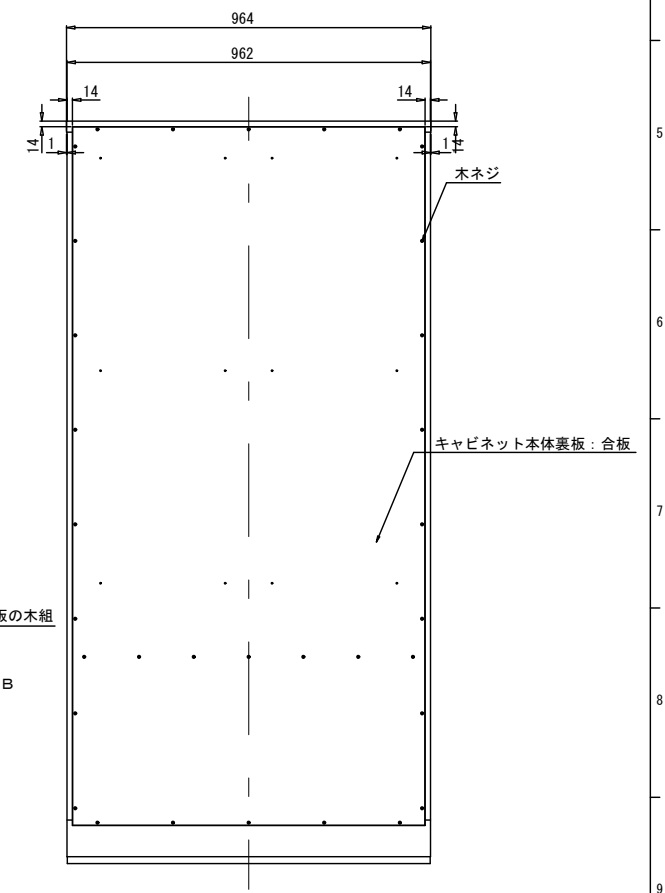
B-B 断面図 S=1/10 (S=1/20)
