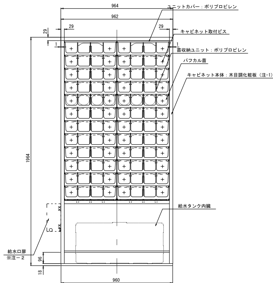
正面図 S=1/10 (S=1/20)
